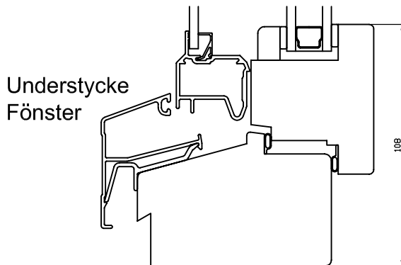
Fig.2 Stor L-profil
