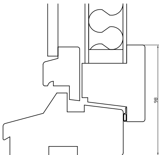
Understycke Dörr
